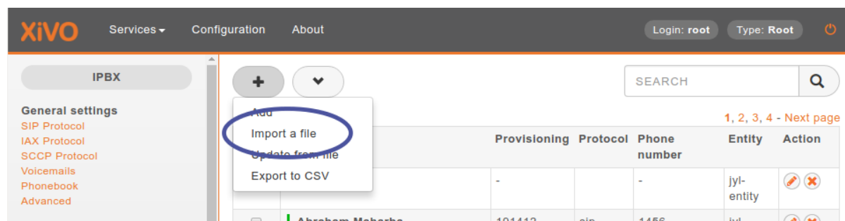
Fig. 45: Import Users
