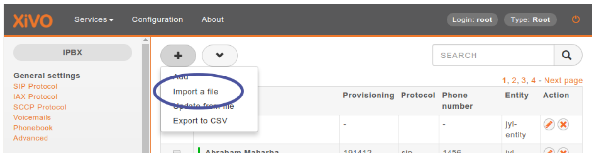
Fig. 45: Import Users
